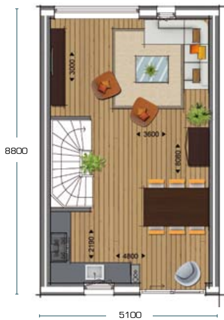
1 e verdieping
