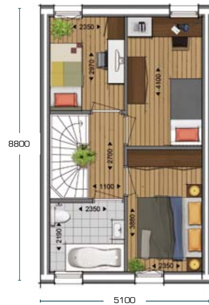
2 e verdieping
