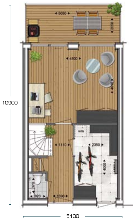
Begane grond
